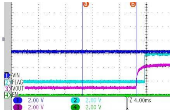
UVLO_H
